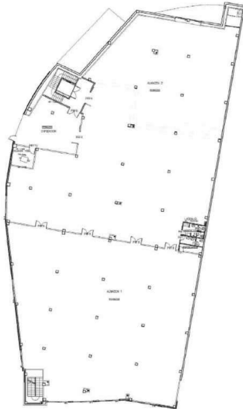
Plano de distribución (planta alta)
