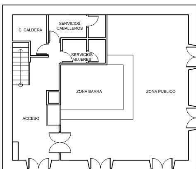
PLANTA BAJA
