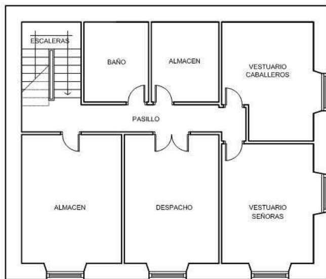
PLANTA SEGUNDA
